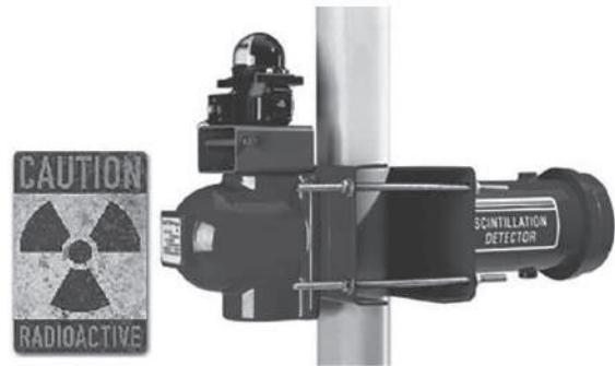
Рис. 1. Радиоизотопный плотномер, установленный на вертикальной стальной трубе с подачей пульпы снизу вверх
